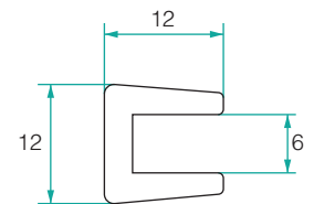
Perfil U 6 mm
